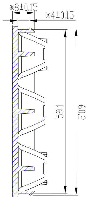
B-B 2:1
